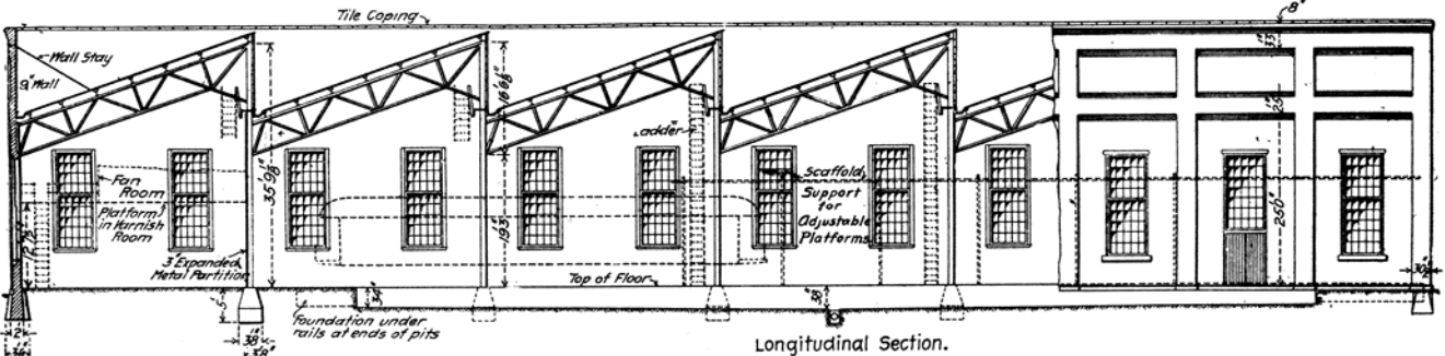
Longitudinal Section.
